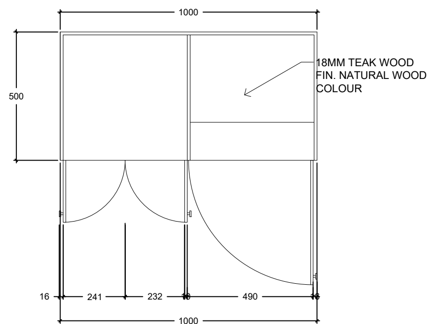
GAMBAR TAMPAK ATAS SCALE 1: 15
