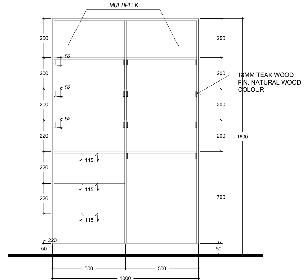
POTONGAN ISI DALAM SCALE 1: 15
