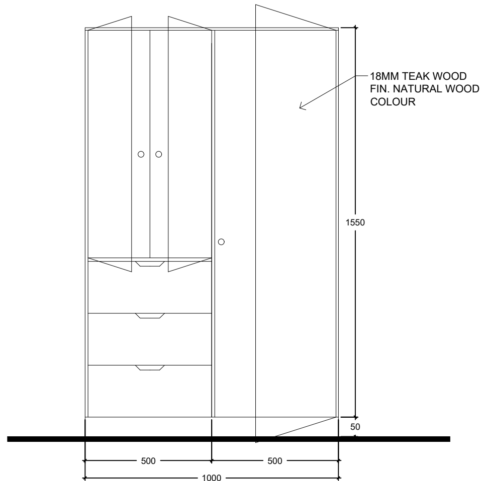
GAMBAR TAMPAK DEPAN SCALE 1: 15
