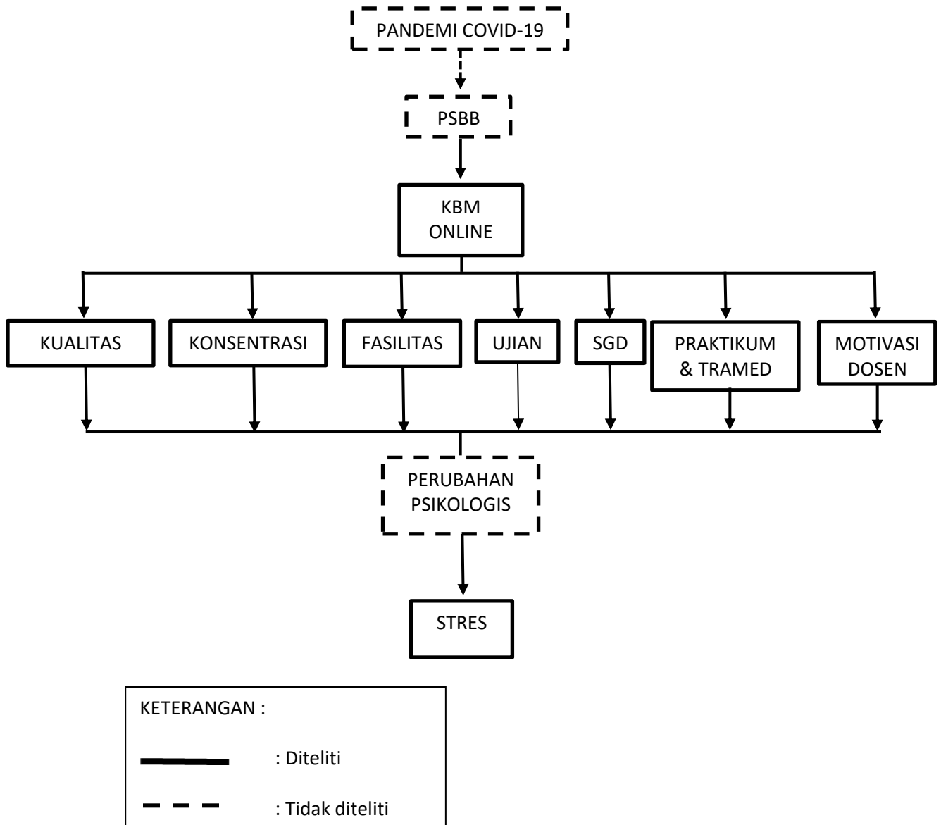
Gambar 3.1 Kerangka Konsep
